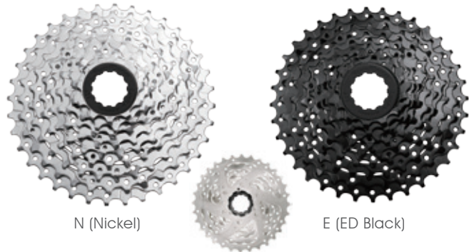
CSM98 9AW 11-36T 9BW 12-36T
